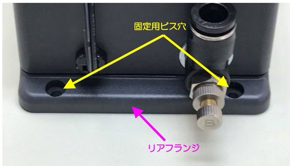
本体固定用フランジ (後側)
